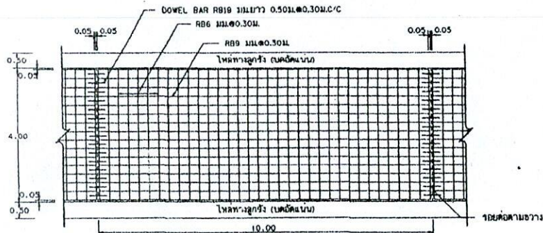
แปลนแสดงการเสริมเหล็กถนน คลส. NOT TO SCALE
